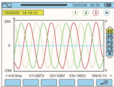
(波形测试界面)
